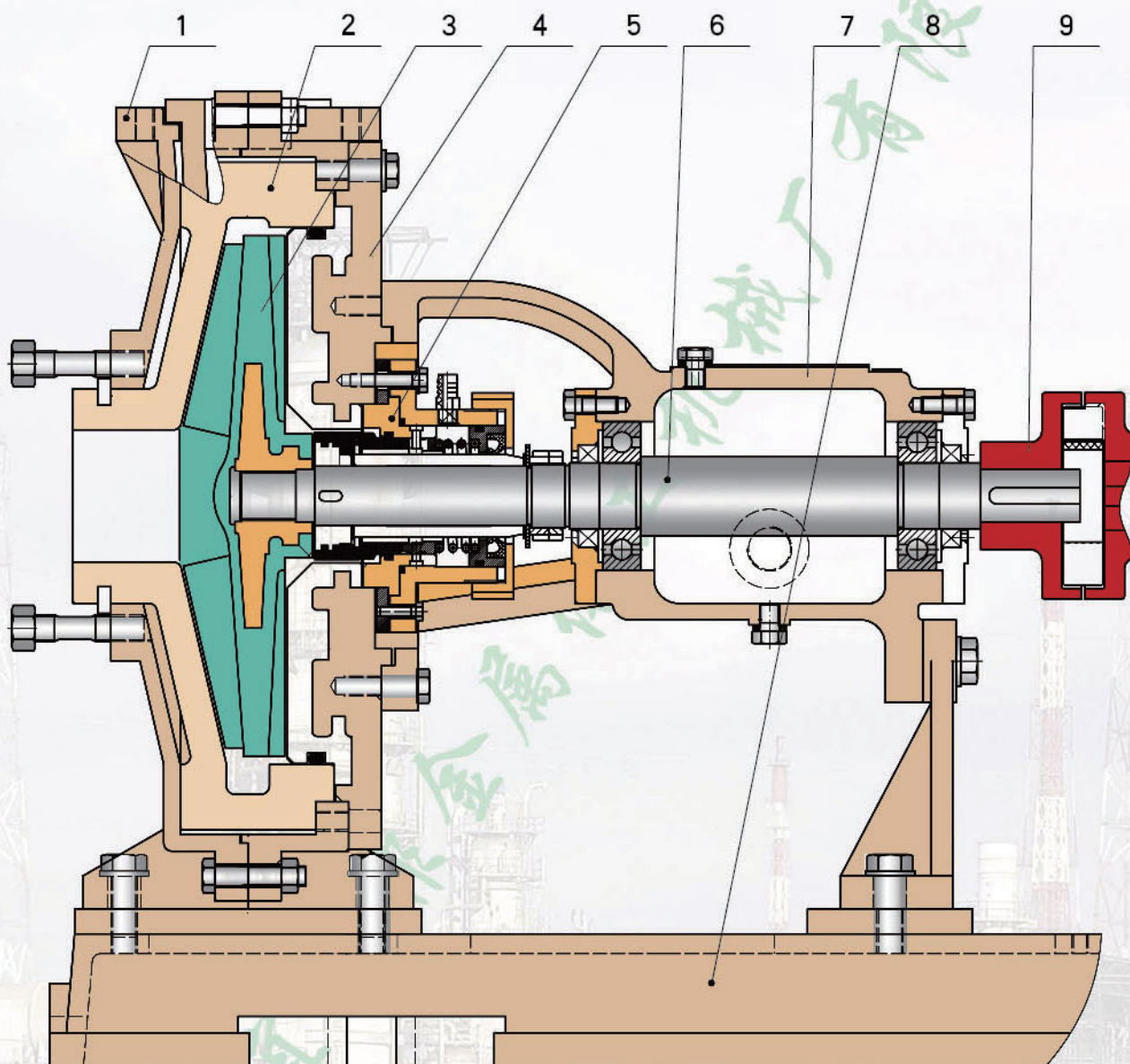
1. 铁泵体 2. 塑泵体 3. 叶轮 4. 泵盖 5. 密封部件 6. 主轴 7. 轴承座 8. 底座 9. 联轴器
